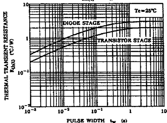
R_{th}(t) - t_w
