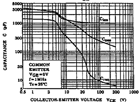
C - V_{CE}
